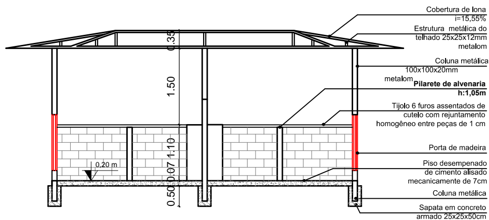
Corte AA Esc. 1:75
