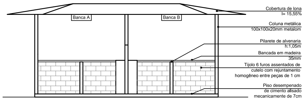
Fachada Esc. 1:75
